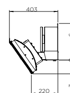
Vue latérale (sans déflecteur de chaleur)
