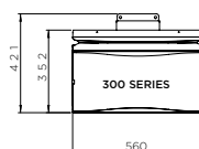
Vue de face (avec déflecteur de chaleur)
