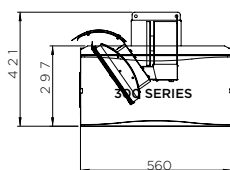
Vue de face (sans déflecteur de chaleur)
